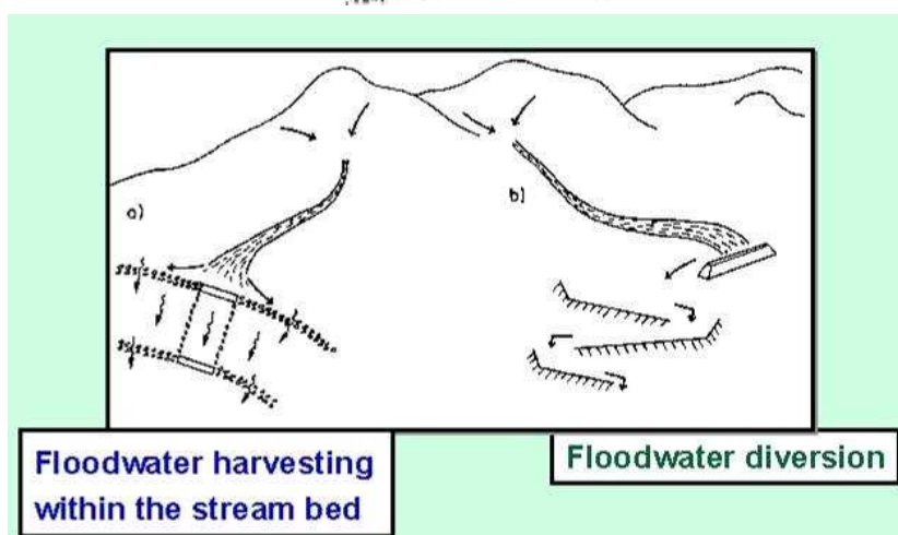
شکل شماره ۷-۱۲- سیستم جمع آوری سیلاب‌ها از بستر رودخانه و پخش سیلاب
