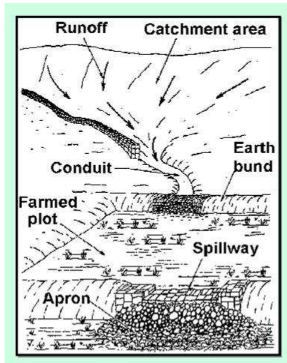
شکل شماره ۷-۱۱- جمع آوری آب به روش سیستم کشت در دامنه تپه‌ها
