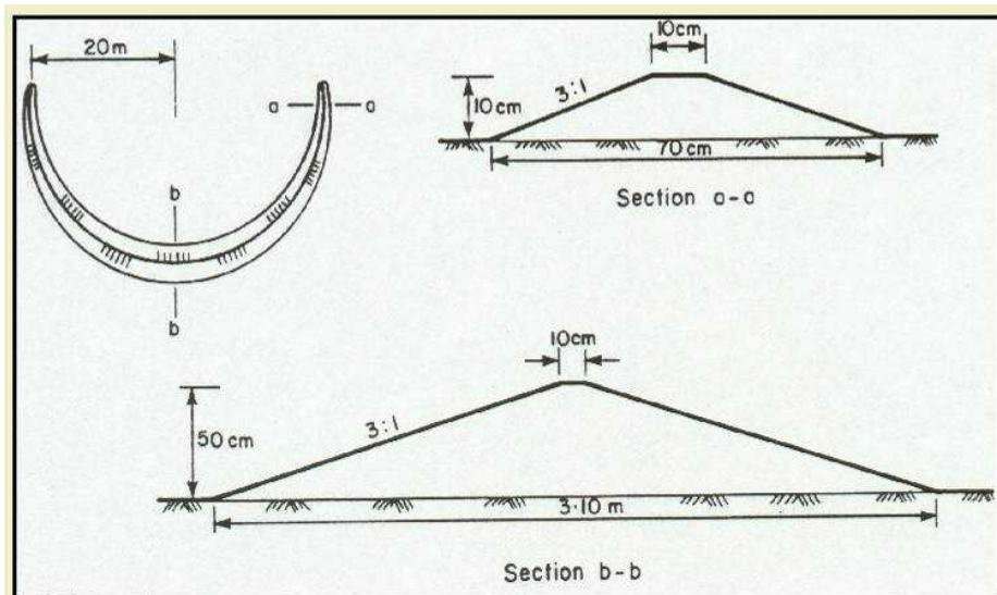
شکل شماره ۷-۵- جمع آوری آب به روش باندهای نیم دایره‌ای
