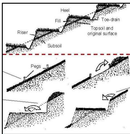
شکل شماره ۷-۴- جمع آوری آب به روش تراس‌های سکویی کنتوری
