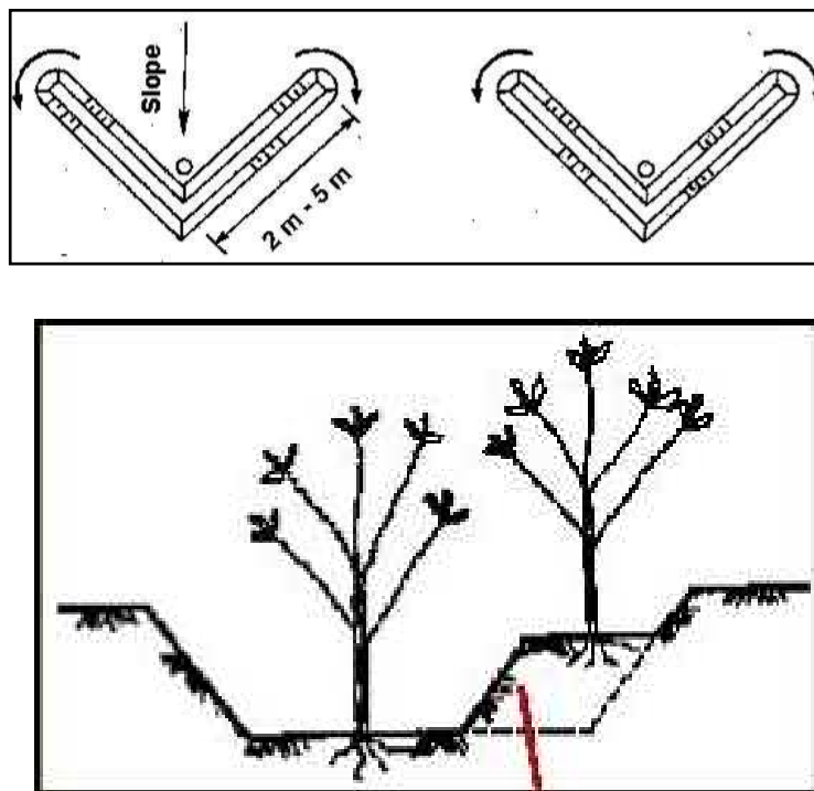
شکل شماره ۷-۶- جمع‌آوری آب به روش باندهای مثلثی
