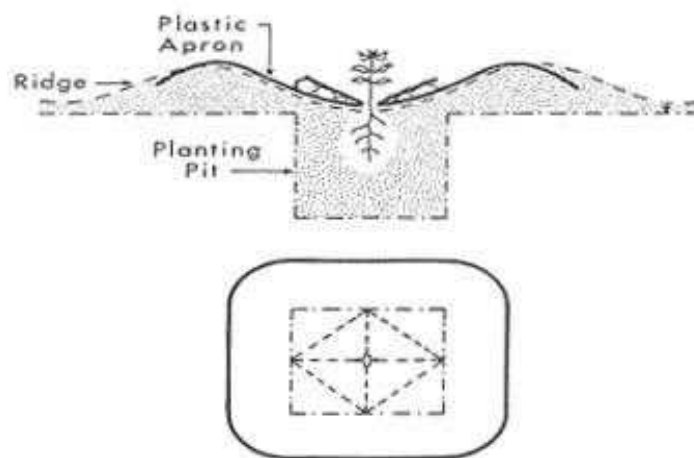
شکل ۷-۱- استفاده از پلاستیک بمنظور افزایش میزان نگهداری آب
