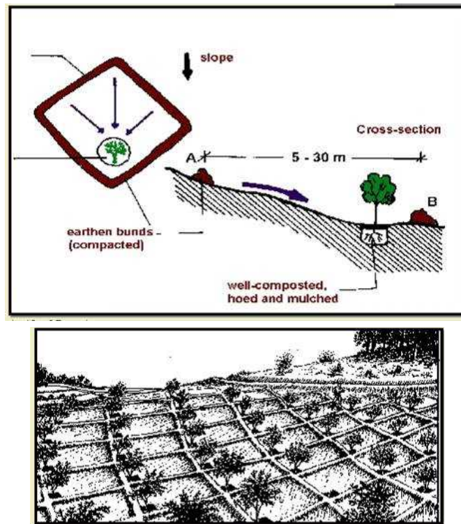
شکل شماره ۷-۹- جمع آوری آب به روش ریزحوضه لوزی شکل
