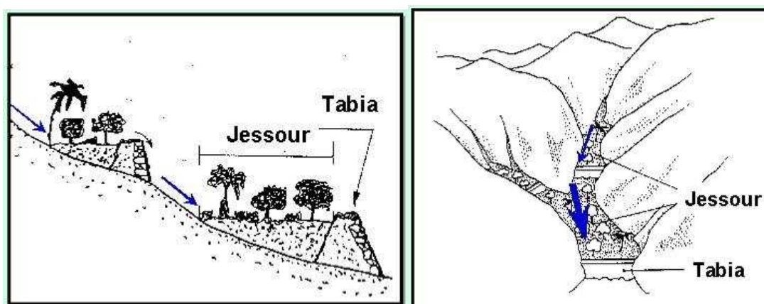
شکل شماره ۷-۱۳- دره بند هلالی یا ژسور
