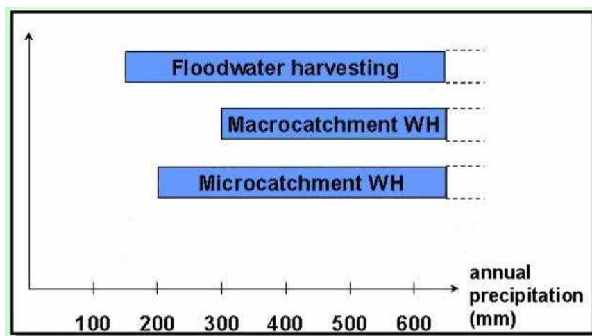
شکل شماره ۷-۱۶- انتخاب نوع سیستم جمع آوری با توجه به میزان بارش سالیانه
