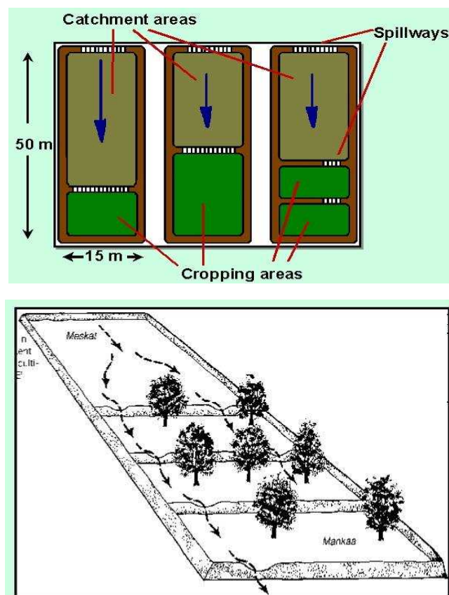
شکل شماره ۷-۸- جمع آوری آب به روش کرتی
